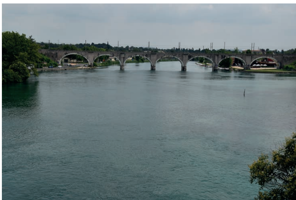
Obr. 19. Výtok rieky Mincio z Gardského jazera v Peschiera del Garda neďaleko pevnosti
