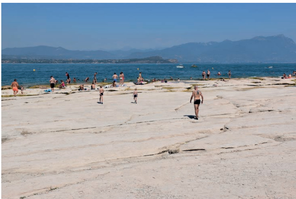
Obr. 18. Pri nízkom vodnom stave Gardského jazera (v roku 2022) v obnaženom skalnom pobreží polostrova Sirmione vidno v jeho ľadovcom vyhladenom povrchu exaráčné ryhy vytvorené blokmi hornín vmrznutých do spodku ľadovca
